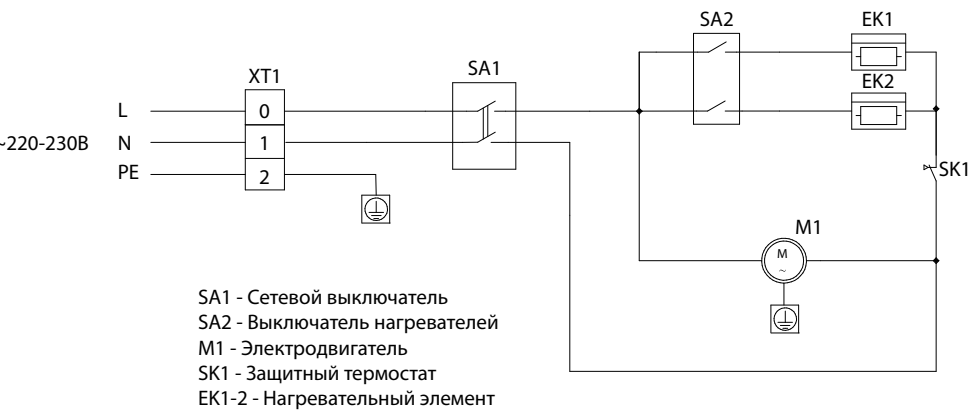
Рис. 2. Электрическая схема принципиальная BIGH-55 F
