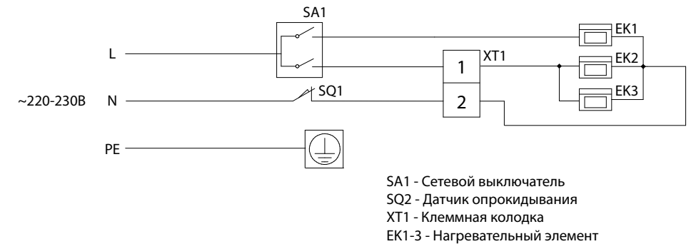
Рис. 1. Электрическая схема принципиальная BIGH-55 H
