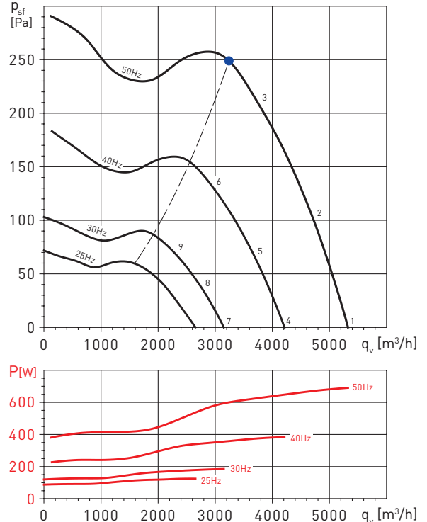
TD-6000/400 TRI
