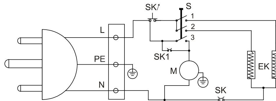
Рис.4. Электрическая схема КЭВ-3С41Е
